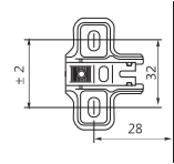
Calço para Dobradiça Rabo Curto SH Base for Short Arm Hinge
