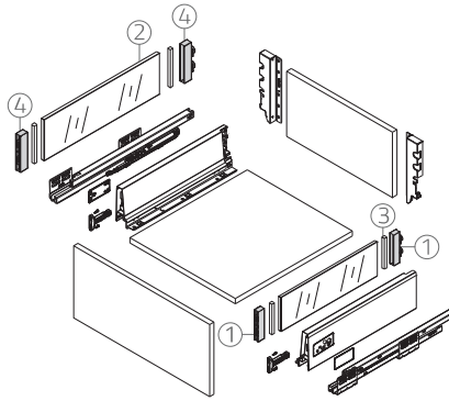
Q57 Redução de Vidro P/ Acrílico Alto DTC DTC Glass Reduction
