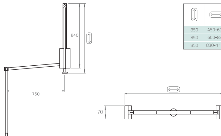
Suporte Basculante para Roupeiro Tilting Support for Wardrobe
