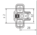
Calço Normal para Dobradiça c/Amort. Blama Normal Base for Blama Soft Close Hinge
